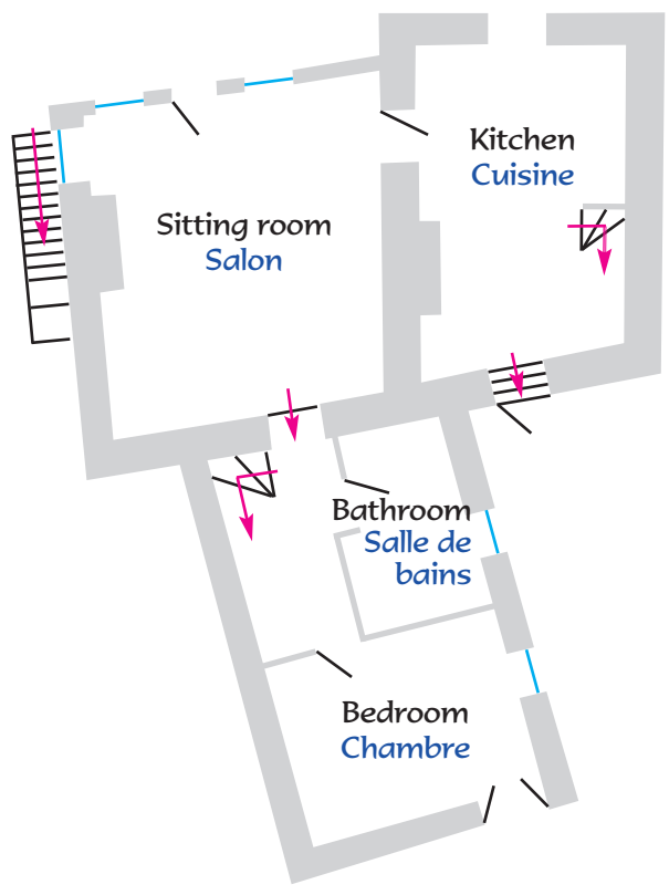
Ground floor plan Plan du rez-de-chaussée
